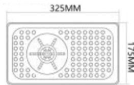
嵌入式洗杯器_S號
