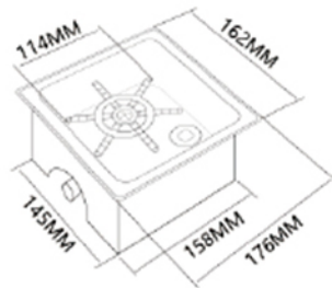
台式洗杯器_XS號
