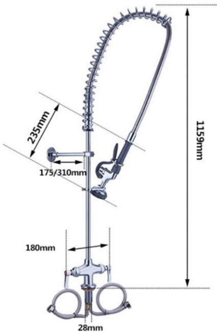
標準型預洗噴槍
