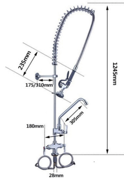
標準型預洗噴槍帶搖擺龍頭
