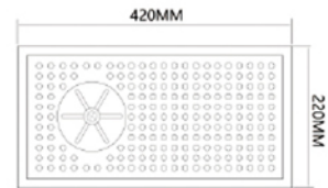
嵌入式洗杯器_M號
