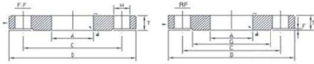
JIS 10kg/cm 2 型 FLANGES
