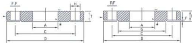
JIS 16kg/cm 2 型 FLANGES
