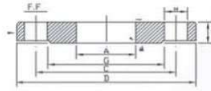
ANSI 125型 FLANGES
