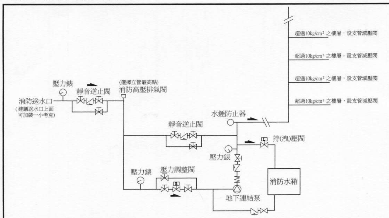
灑水配管參考圖
