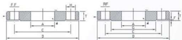
ANSI 300型 FLANGES
