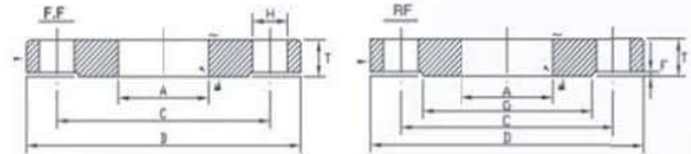
ANSI 150型 FLANGES
