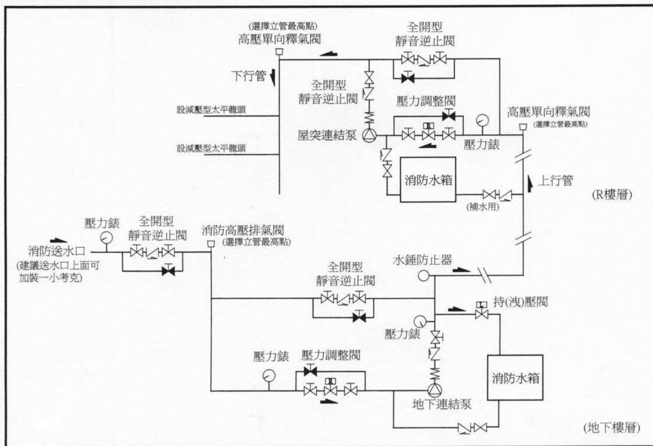
連結配管參考圖
