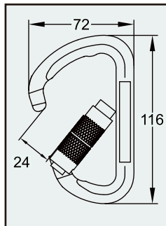
D1 Carabiner CBRAD1-ALF-004
