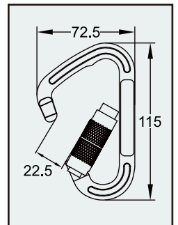
D1 Carabiner CBRAD1-ALF-001
