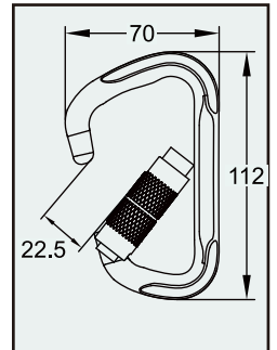
D1 Carabiner CBRAD1-F-002
